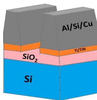
Rajah 1. Gambaran elektrod daripada AlSiCu yang mempunyai keserongan sebanyak 70^\circ .
